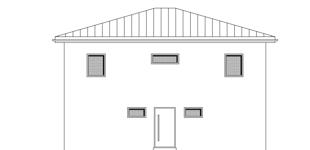
Ansicht Norden
